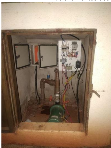
Figura 17 a, b e c – Figuras ilustrando o quadro do comando inserido no local de acionamento da bomba e acionamentos dos aspersores no jardim.
