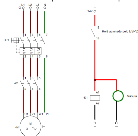
Figura 16 – Esquema de acionamento de potência e comando para acionamento do motor e válvulas.
