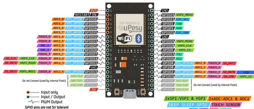
Figura 2 – Microcontrolador utilizado com mapa dos pinos. ESP32 Wroom DevKit Full Pinout
